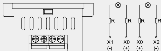
4、四个接线柱（无公共端，中间两个接线柱为正极）
