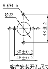
手柄带钥匙型 LW39-16A YS-□-□/□□
