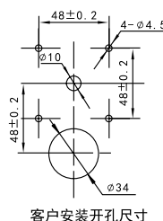
面板带钥匙型 LW39-16A YM-□-□/□□□
