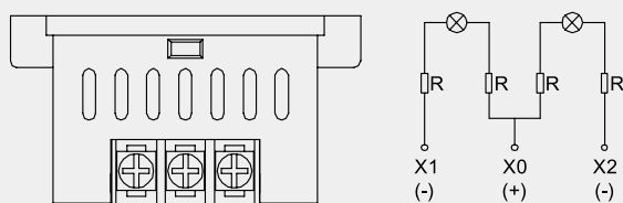
2、三个接线柱（公共端为正极）
