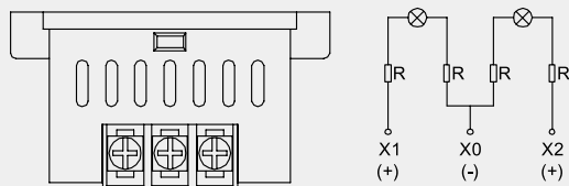
1、三个接线柱（公共端为负极）
