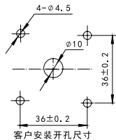
一般型 LW39-16B-□ - □ / □□□
