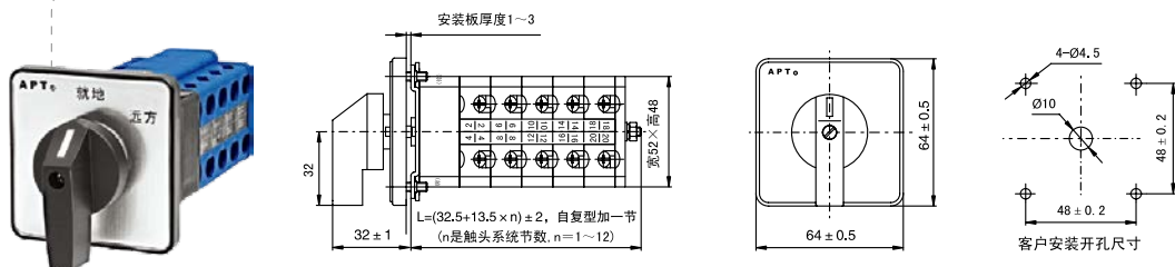
一般型 LW39-25-□-□/□□□
