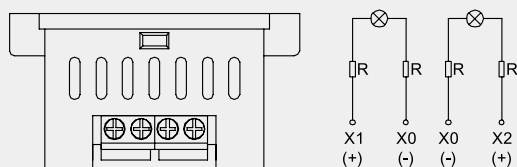
3、四个接线柱（无公共端，中间两个接线柱为负极）
