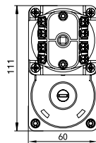
面板带钥匙型 LW39-16A YM-□-□/□□□
