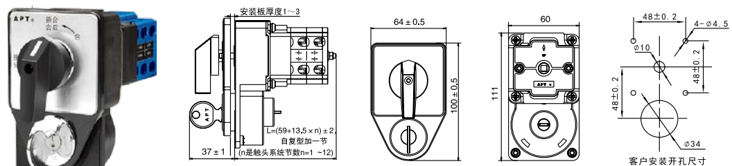
面板带钥匙型 LW39-25 YM-□-□/□□□
