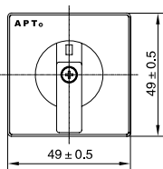
底座安装型 LW39-16B M - □ - □ / □□□
